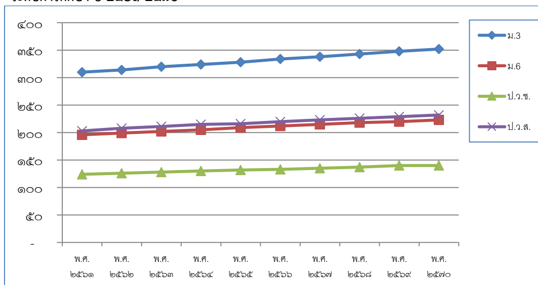
แผนภูมิที่ ๑๕ ผลการคาดการณ์การผู้สำเร็จการศึกษาและพร้อมที่จะเข้าสู่ตลาดแรงงานของประเทศ จำแนกตามระดับการศึกษา ปี ๒๕๖๑-๒๕๗๐
